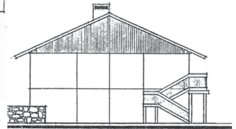
БОКОВОЙ ФАСАД.
