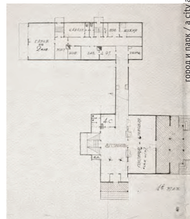
^ Рис. 3. Проект дома отдыха штаба РККА. План первого этажа. Архитекторы В. И. Пилявский, Е. Б. Серебряков. 1932 (ЦГАЛИ СПб. Ф. Р.-453. Оп. 1. Д. 172. Л. 3)
