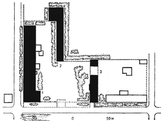
^ Рис.11. Генплан-схема усадьбы Бутиных. Обмер Н. П. Крадина
