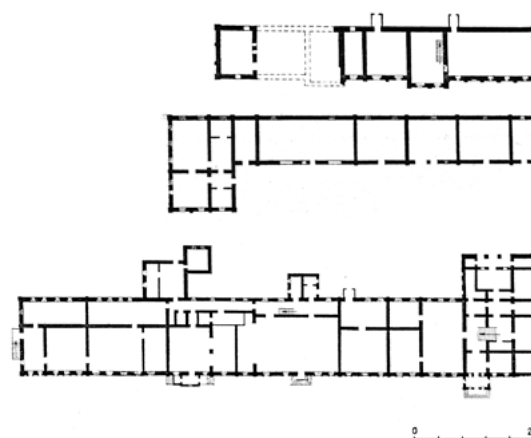
< Рис.14. Планы зданий дворцового комплекса: дворец, водонапорная башня с оранжереей, каретные ряды. Обмеры Н. П. Крадина
