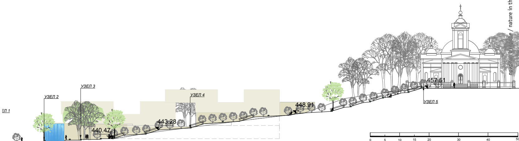
^ Разрез по оси лестницы и двум площадям
